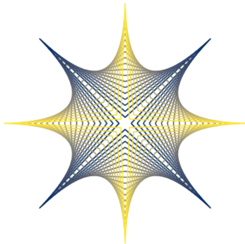
cividis
