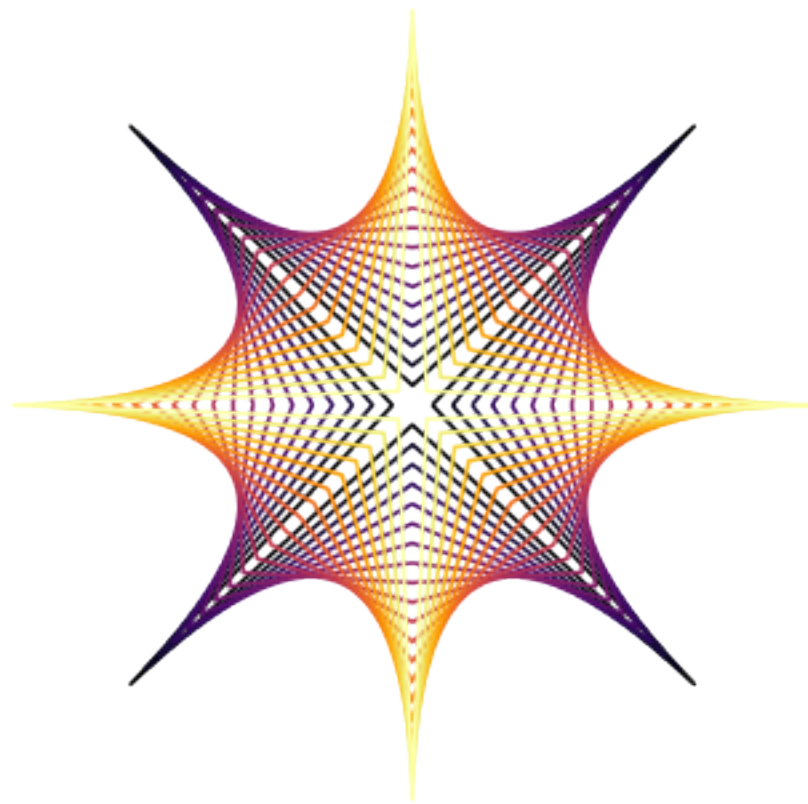
inferno
