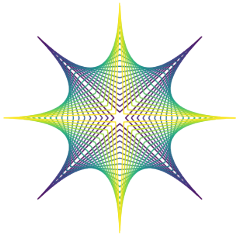
viridis
